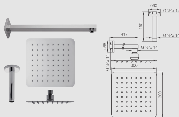
FR126.05.1.0 Ducha cuadrada de 300 mm. con brazos De pared y de techo. AI-BB-BG-BK-BN PB-PG-PN-SGR
