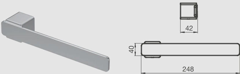
FV163/J5 Toallero corto. PC-FB
