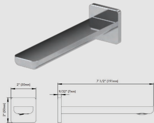
FV103/J5.17.0 Pico de bañera de pared con conexión hembra NPT de 1/2. PC-FB
