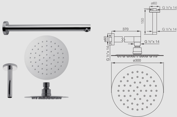
FR126.04.1.0 Ducha redonda de 300 mm. con brazos De pared y de techo. AI-BB-BG-BK-BN PB-PG-PN-SGR
