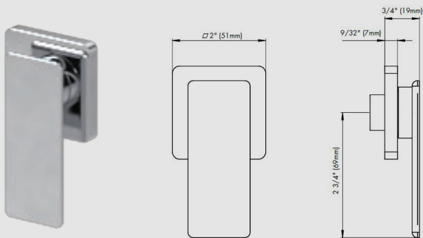
FV480/J5.0 Llave de paso, solo vista. PC-FB
